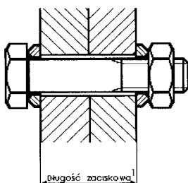
zestaw śrubowy HV po zmontowaniu БОЛТ HV после монтажа / screw HV set after assembling
